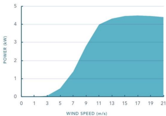
VERMOGENSCURVE
