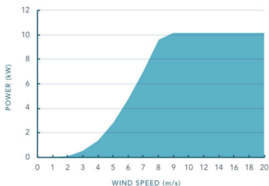
VERMOGENSCURVE
